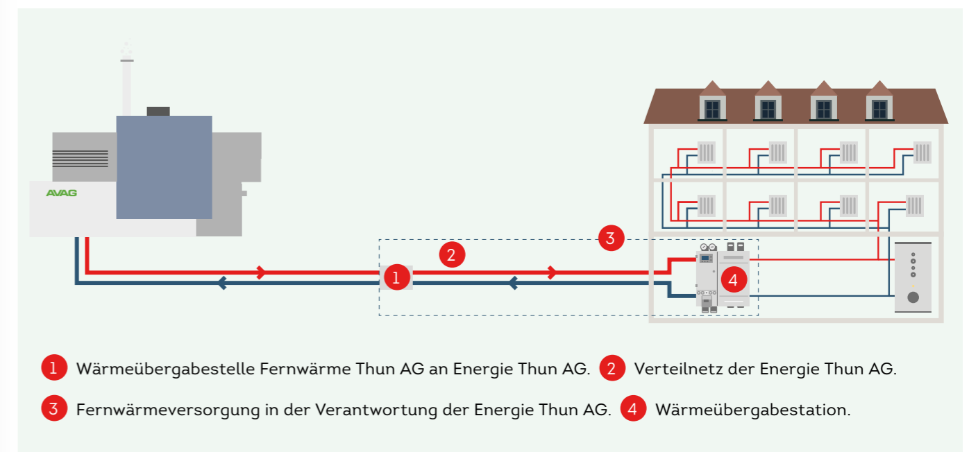
Weg der Fernwärme kurz erklärt.
